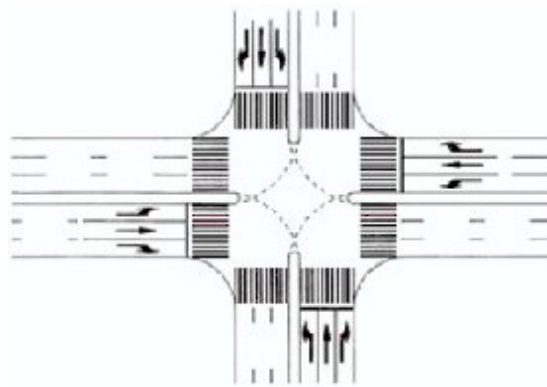
Marcaj pentru spații înguste
