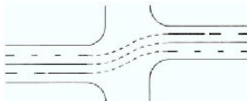
Marcaj de ghidare la traversarea unei intersecții
